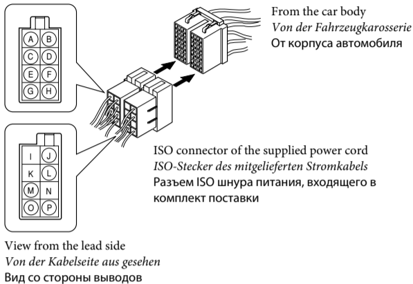
Original wiring / Original verdrahtung / Исходная схема соединений
