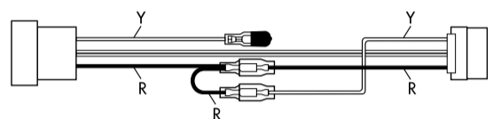
Modified wiring 2 / Modifizierte Verdrahtung 2 / Преобразованная схема соединений 2
